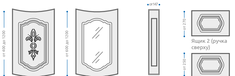
Радиусный фасад
